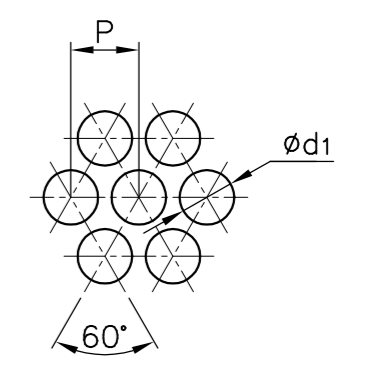
パンチングプレート 詳細
